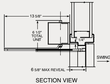
Hollow Metal Door Shown
