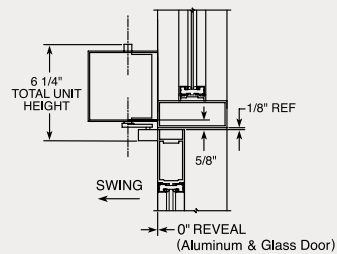
Aluminum & Glass Door Shown
