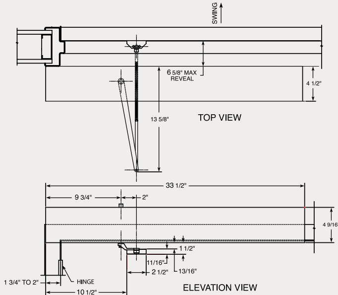
Hollow Metal Door Shown
