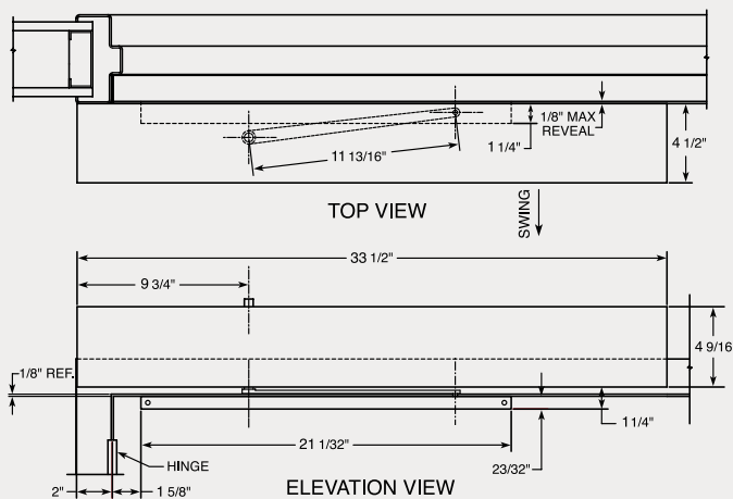
Aluminum & Glass Door Shown
